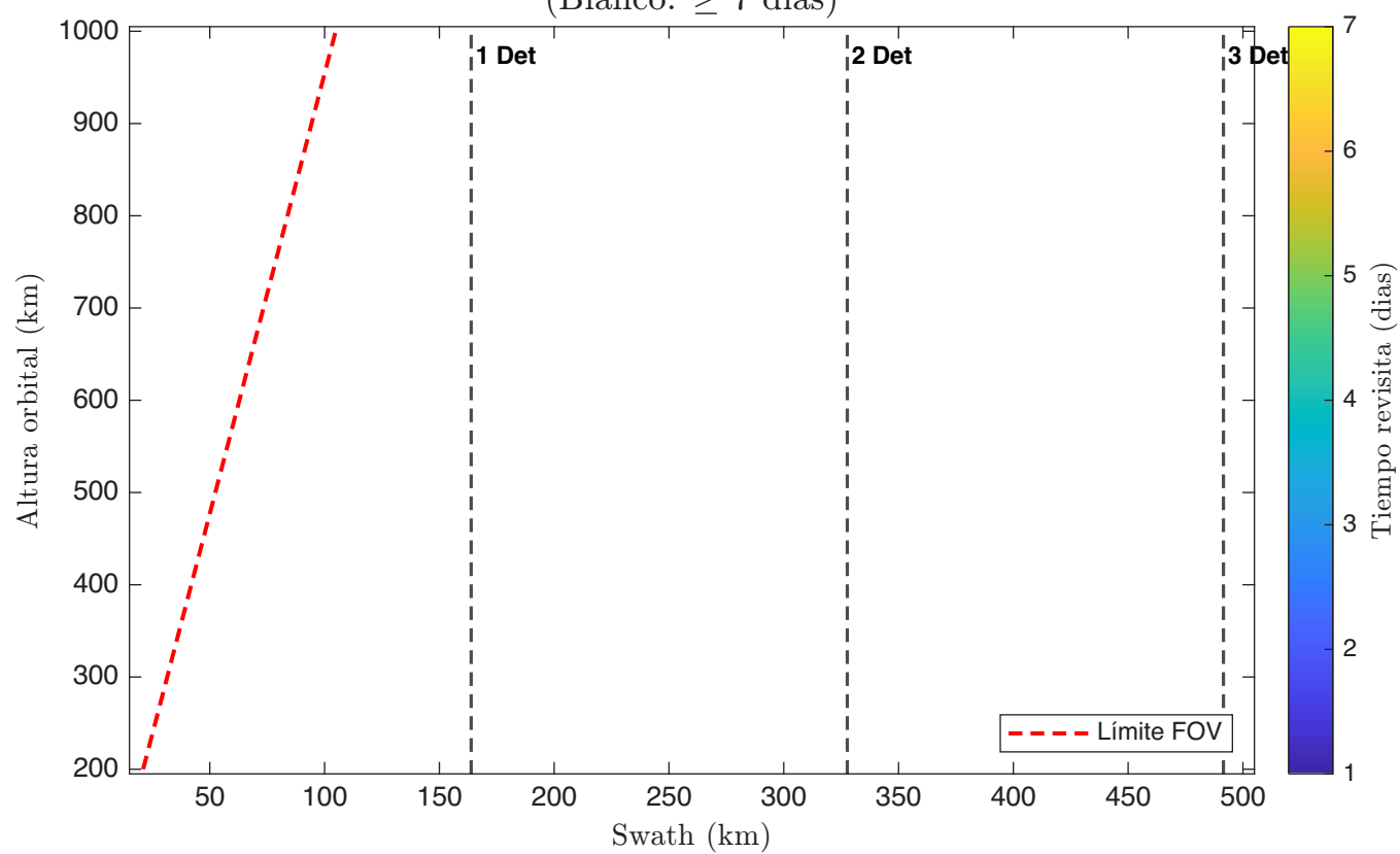
Tiempo Revisita - 2 Satellite(s); 2 Telescopio(s): Cassegrain; Detector 2 (Blanco: \geq 7 dias)
